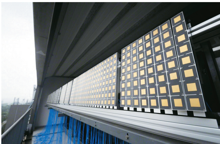
紫金山实验室大规模 MIMO 天线阵列
